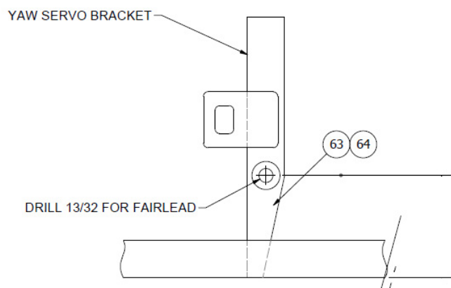
SECTION AF
