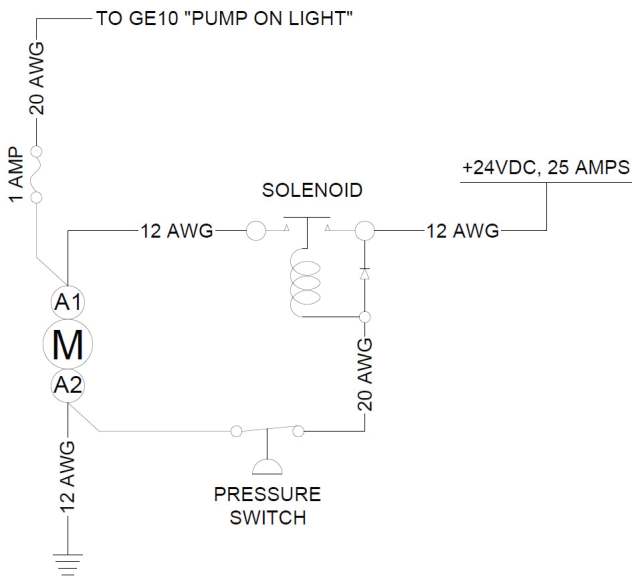
3 LUG SOLENOID ELECTRICAL SCHEMATIC
