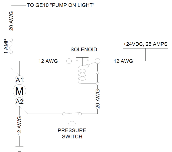
4 LUG SOLENOID ELECTRICAL SCHEMATIC
